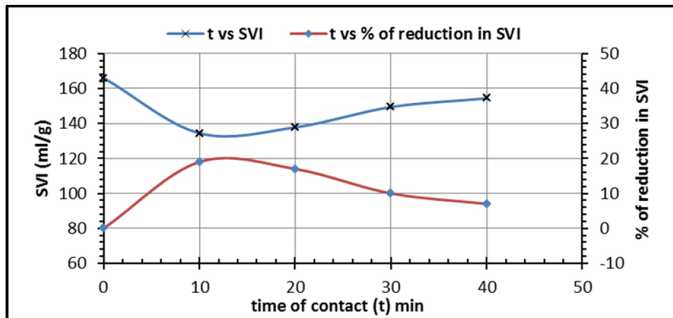
الشكل (6): علاقة زمن التعريض مع (SVI) والنسبة المئوية للانخفاض لـ (SVI) عند التردد (44KHz)
