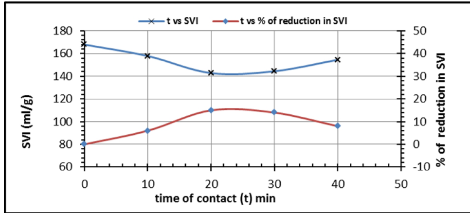
الشكل (5): علاقة زمن التعريض مع (SVI) والنسبة المئوية للانخفاض (SVI) عند التردد (31KHz)
