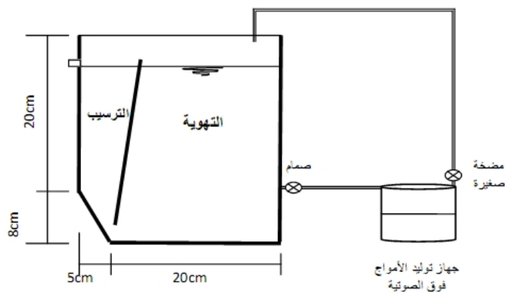
الشكل (2): المنظومة الاختبارية
