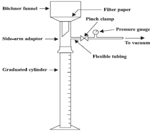
الشكل(3): جهاز قياس المقاومة النوعية للحماة للاحتفاظ بالماء
