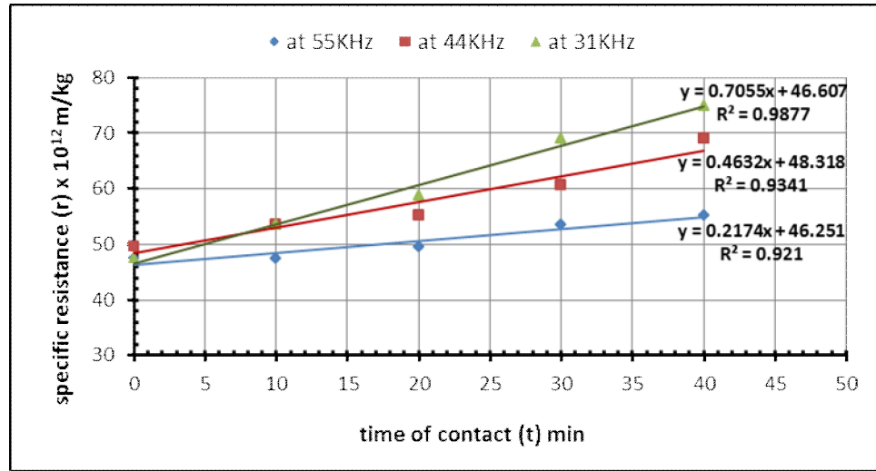
الشكل (9): تأثير زمن التعريض على المقاومة النوعية للحماية للاحتفاظ بالماء عند الترددات المدروسة
