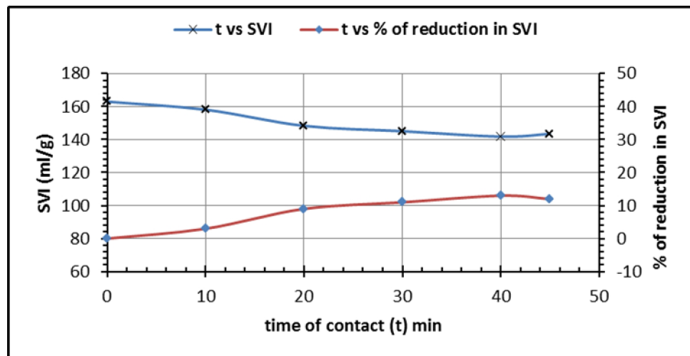
الشكل (7): علاقة زمن التعريض مع (SVI) والنسبة المئوية للانخفاض لـ (SVI) عند التردد (55KHz)
